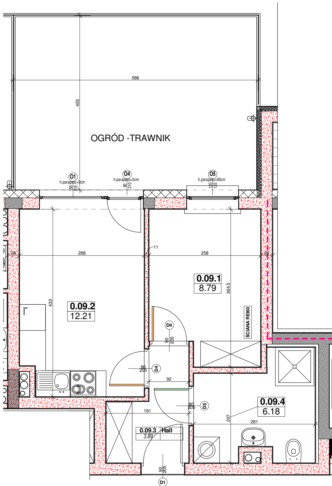
1 Lokal M09 1 : 50
