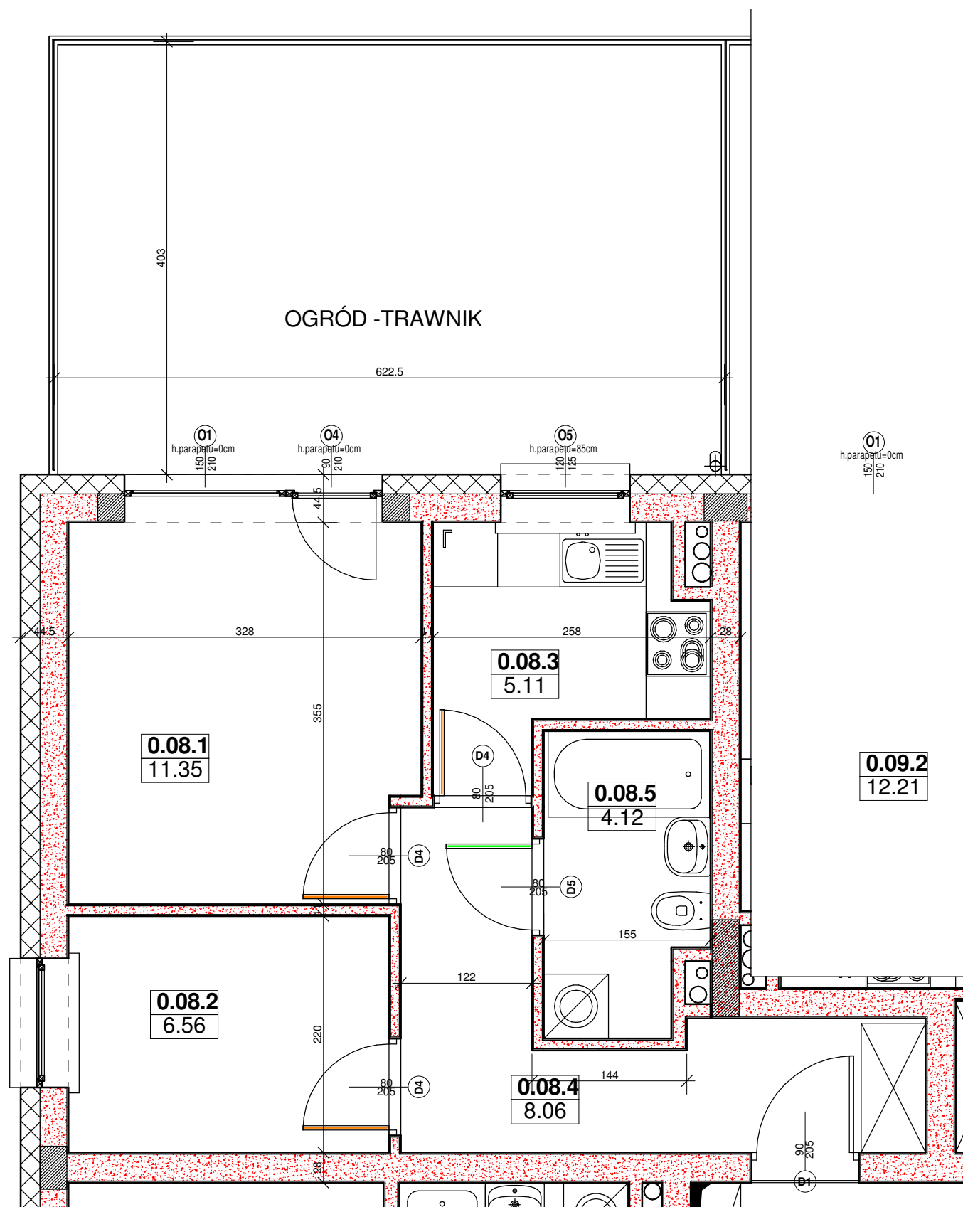
1 Lokal M08 1 : 50
