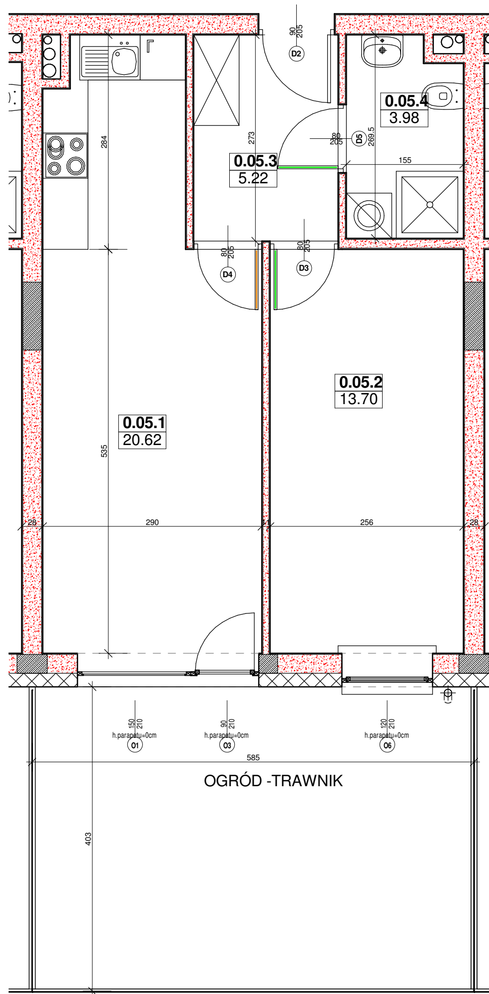
1 Lokal M05 1 : 50
