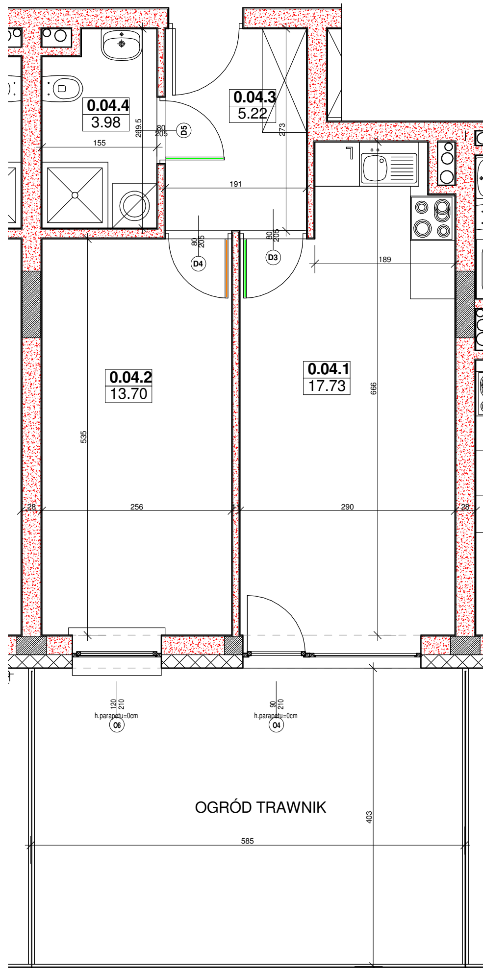
1 Lokal M04 1 : 50
