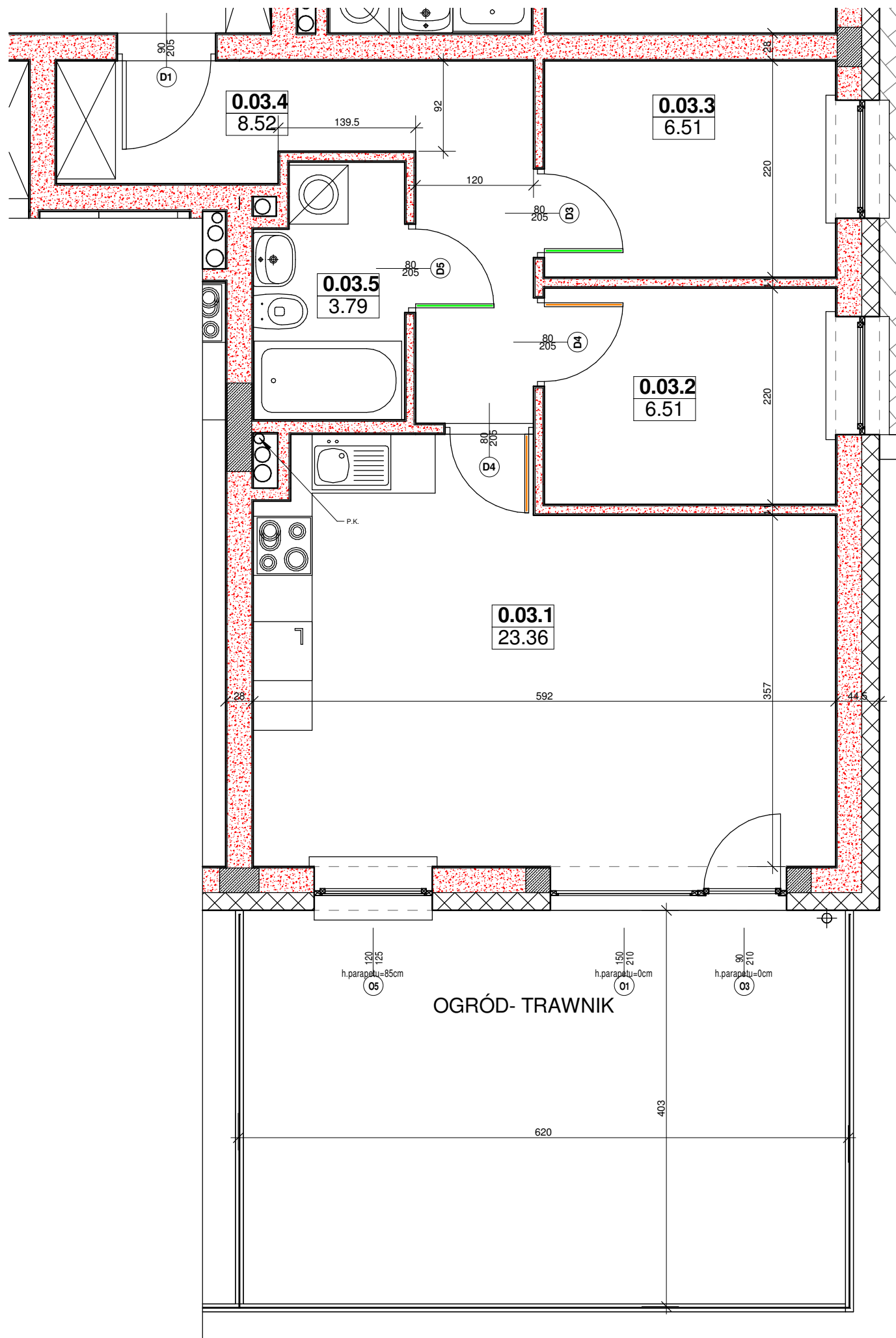
1 Lokal M03 1 : 50
