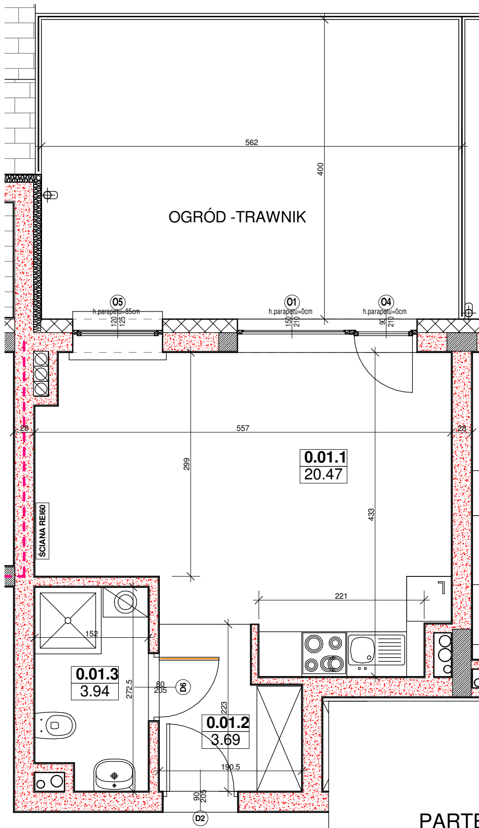
1 Lokal M01 1 : 50
